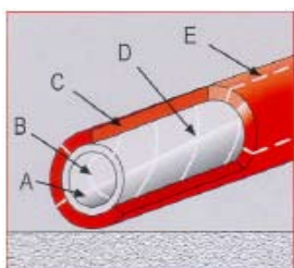
Obr.1 Rez injektážnou hadicou MASTERFLEX® 900 typ 3
